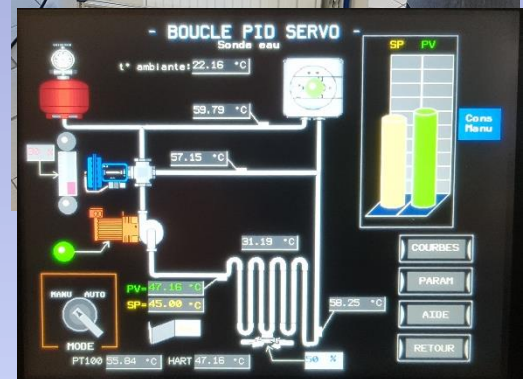
Banc de chauffage + Supervision
